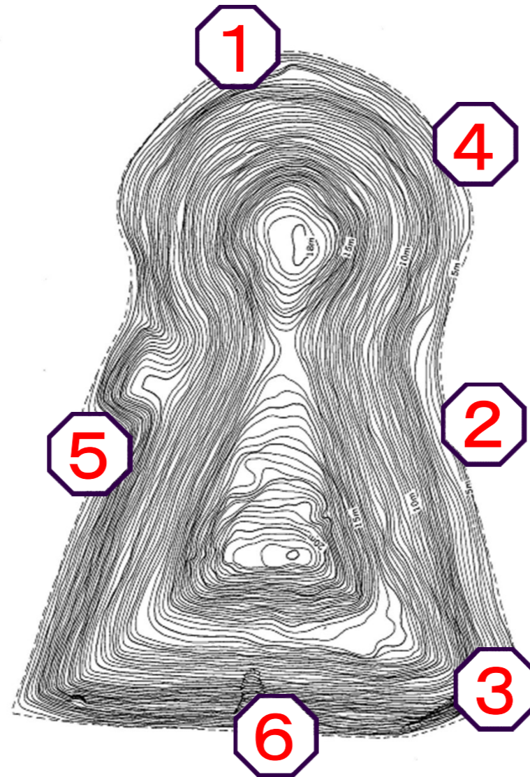
【断夫山古墳測量図】
